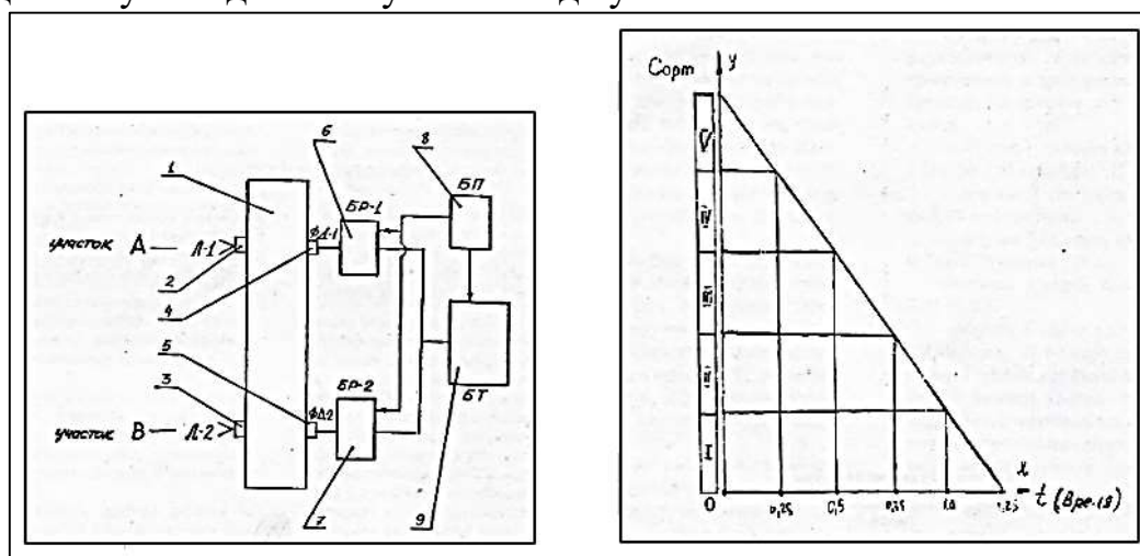
Рисунок 4. - Принципиальная схема прибора для определения сорта хлопка-сырца в полевых условиях и тарифовочный график определения сорта летучки волокна
