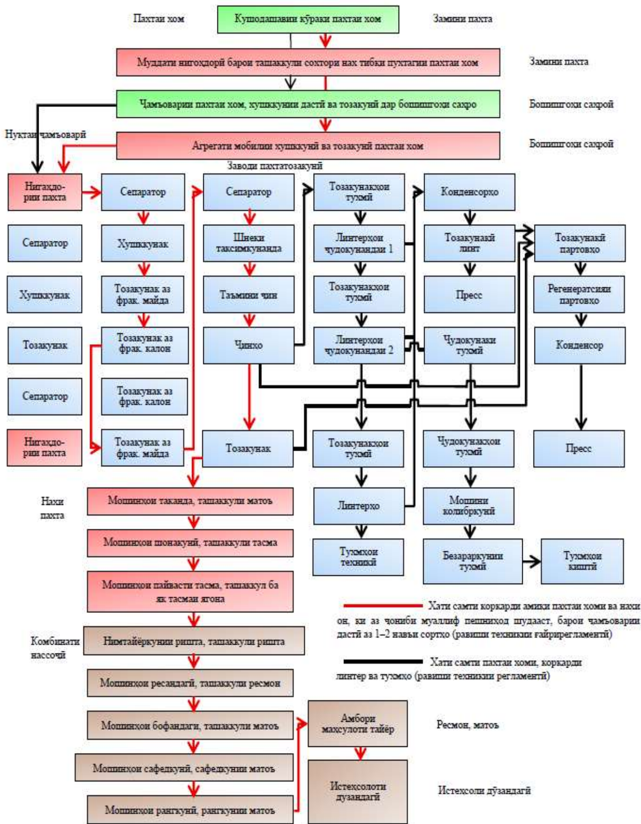
Расми 2. - Нақшаи пешниҳодшудаи ҷараёни технологияи коркарди амиқи механикӣ пахтаи хом ва навъҳои миёнаҳаҷм дар Ҷумҳурии Тоҷикистон (танзимнашаванда) Манбаъ: таҳияи асли
