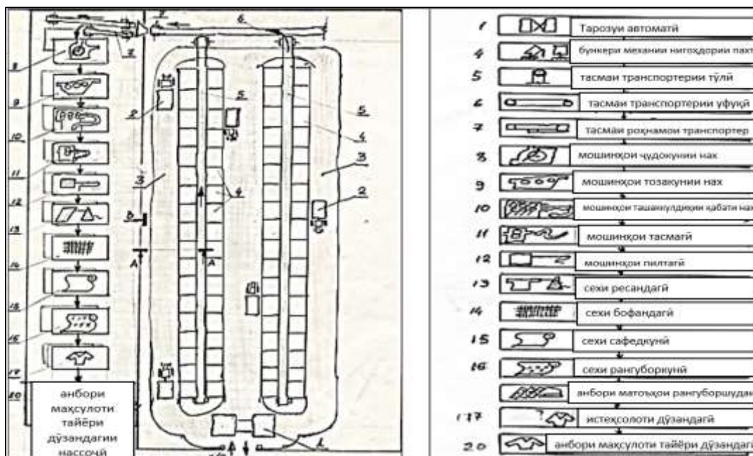
Расми 6. - Нақшаи ҳаракати пахта, раванди технологияи коркарди амиқи пахтаи хом ва нах (механикӣ)
