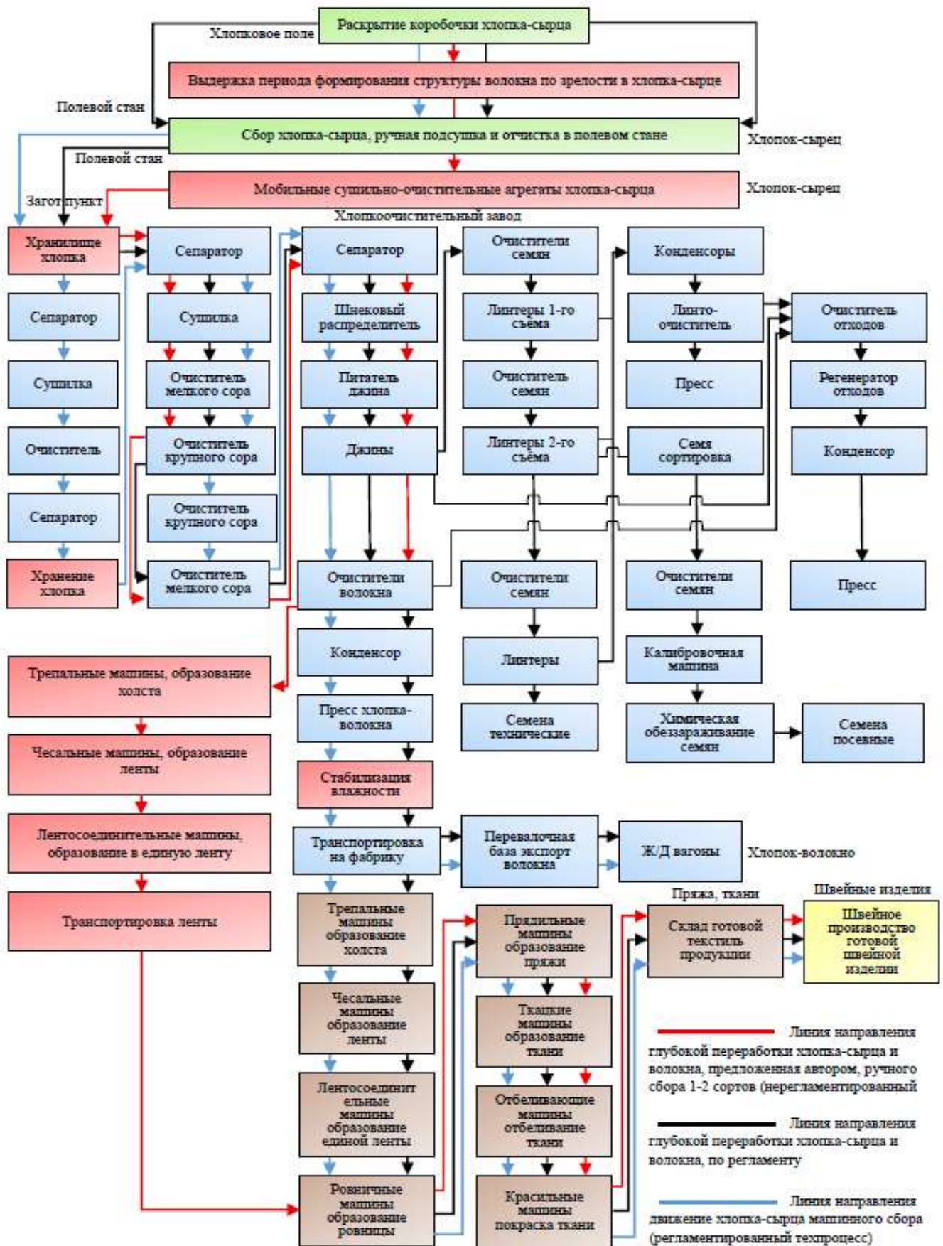
Рисунок 3. - Сравнительная схема технологического процесса глубокой механической переработки хлопца-сырца и волокна средневолокнистых сортов в Республике Таджикистан (регламентированная и нерегламентированная)
