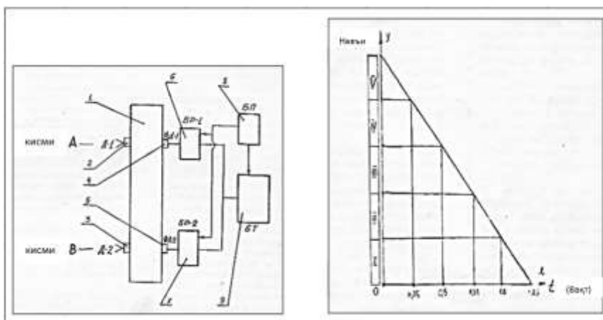
Расми 4.- Диаграммаи нақшавии дастгоҳ барои муайян кардани навъи пахтаи хом дар саҳро бо истифодаи диаграммаи мувофиқақунандаи махсус
