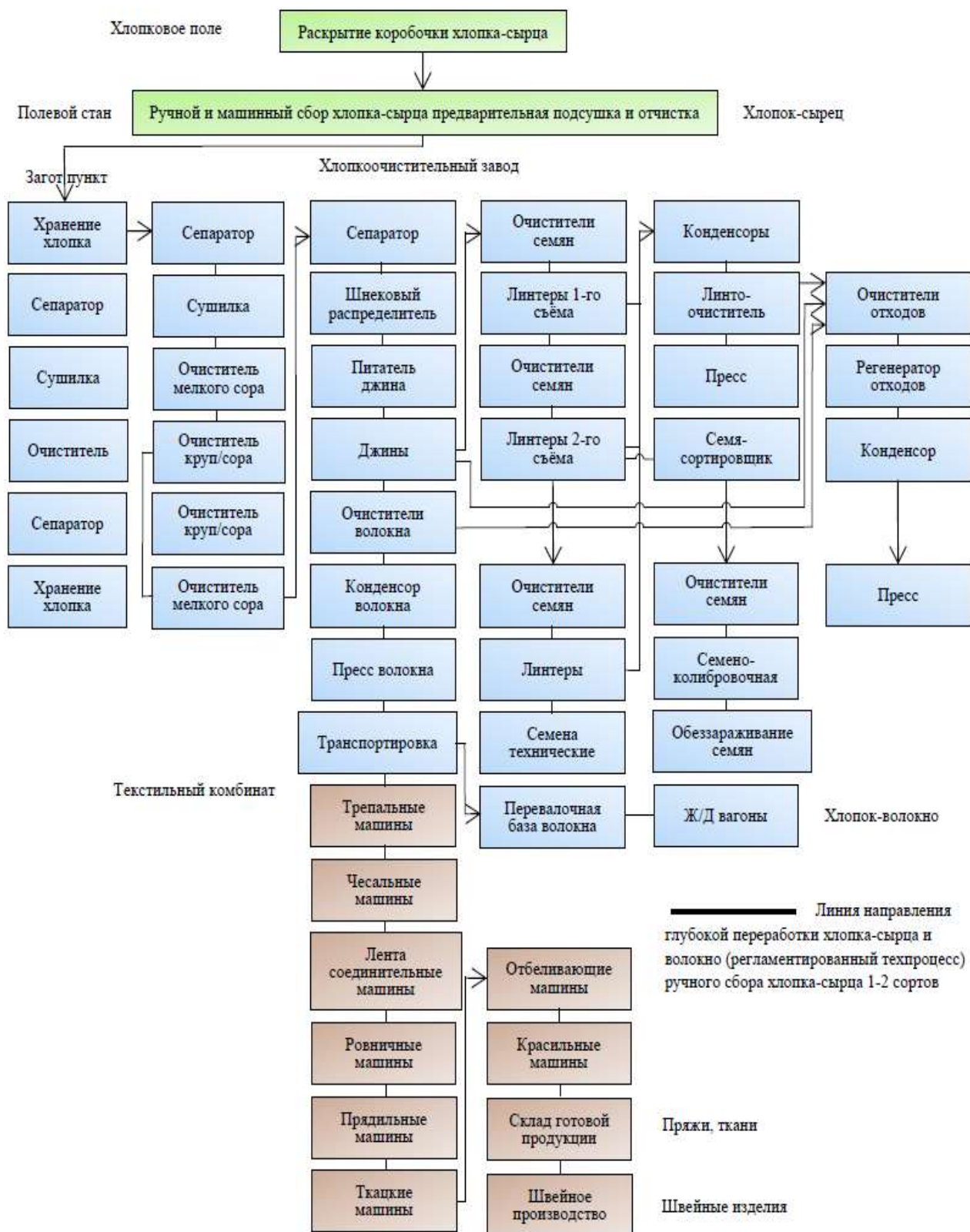
Рисунок 1. - Схема регламентированного технологического процесса глубокой механической переработки хлопка-сырца и волокна средневолокнистых сортов в Республике Таджикистан для ручного сбора хлопка-сырца
