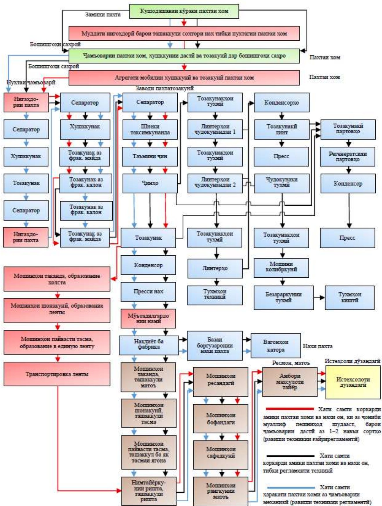
Расми 3. - Диаграммаи муқоисавии раванди технологияи коркарди амиқи механикии пахтаи хом ва нах барои навъи пахтаи миёнаҳаҷм дар Ҷумҳурии Тоҷикистон (танзимшаванда ва танзимнашаванда)
