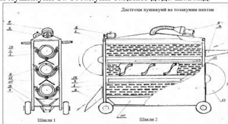
Расми 5. - Дастгоҳи хушккунӣ ва тозакунии пахтаи хом ва нах.
