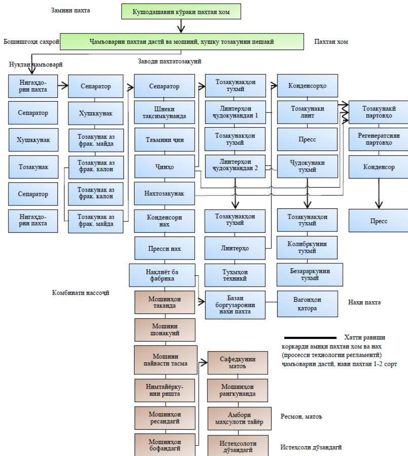
Расми 1. - Нақшаи раванди технологияи танзимшаванда барои коркарди амиқи механикии навъҳои пахтаи хоми миёнаҳа дар Ҷумҳурии Тоҷикистон барои пахтаи хоми дасти чамъовардашуда
