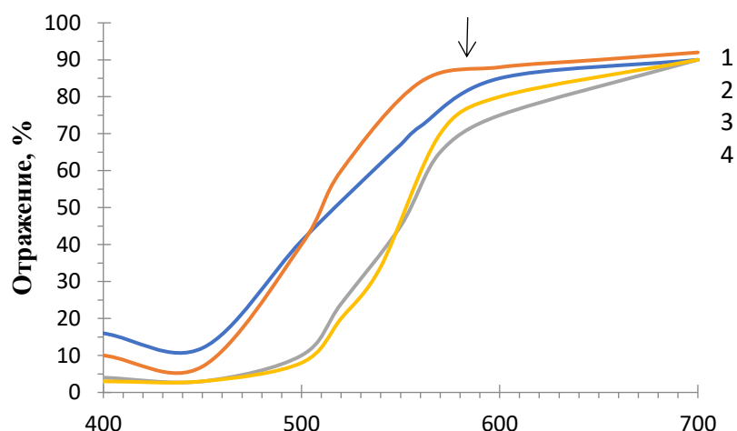
Рисунок 7 – Спектры отражения хлопчатобумажной сатины, различных способов подготовки с печатью (капельный метод) активными чернилами Orange Kiian Digital (где: 1- двухстадийное беление, 2- печать пигментами, 3- расшлихтовка и одностадийное беление, 4- биоотварка).
