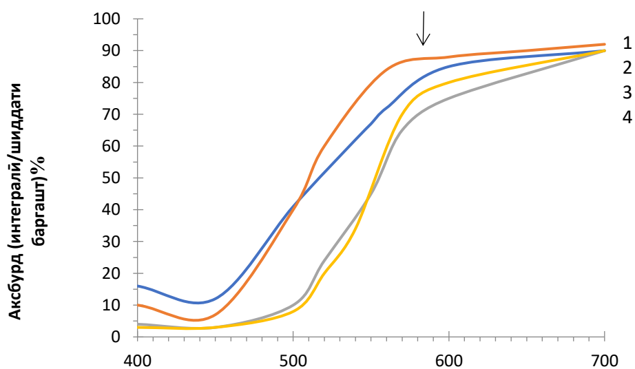
Расми 7 – Спектрҳои аксбурди сатини пахтагӣ бо усулҳои гуногуни оmodасозӣ ва чопи рақамӣ (усули қатрагӣ) бо маҳлули чопии ранги фаъл Orange Kiian Digital, ки дар он: 1 – сафедкунӣ ду марҳалавӣ, 2 – чоп бо пигментҳо, 3 – беширешгардонӣ ва сафедкунӣ якмарҳалавӣ, 4 – биокоркард (ферментативӣ).
