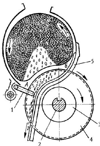
Рис.1. Схема процесса пыльного джинирования хлопка-сырца.
