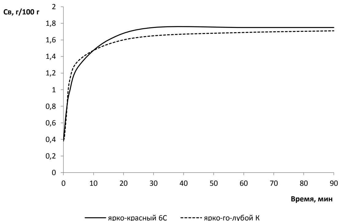
Рисунок.1. Кинетические кривые сорбции активных красителей ярко-красного 6С (1) и ярко-голубого К (К)
