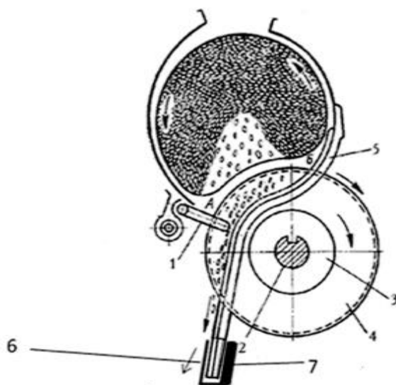
Рис. 2. Рекомендуемая схема процесса пыльного джинирования хлопка-сырца.
